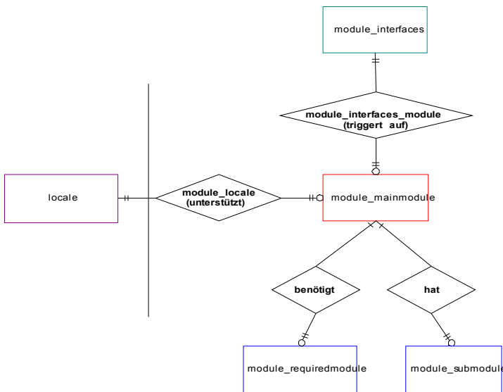
PhPepperShop Modulsystem (ER-Diagramm)
